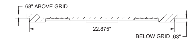
SECTION A-A
