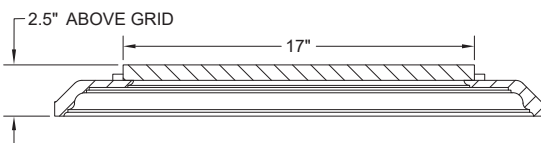
SECTION A-A
