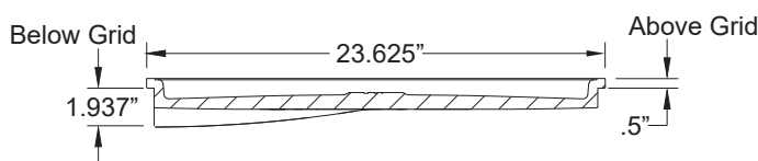
SECTION A-A
